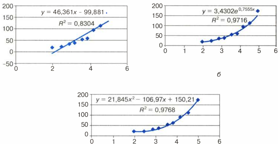
Рис. 3.5. Три функции, построенные по МНК
